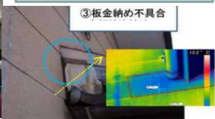
(赤外線画像例)
